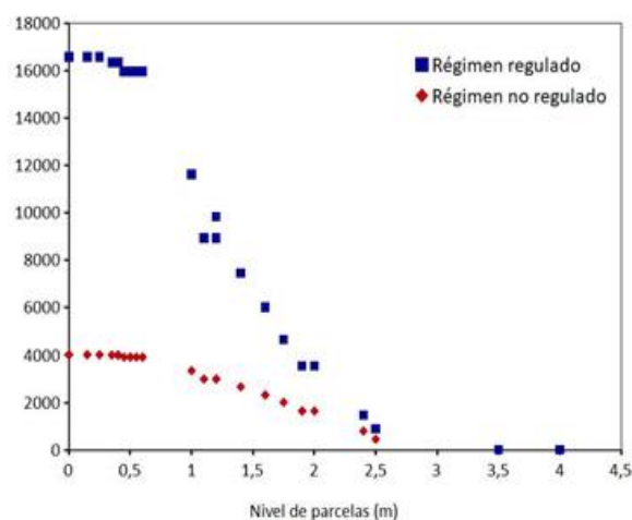
Fig.1. Frecuencia de los niveles de inundación del río Limay, previo y posterior a su regulación.
