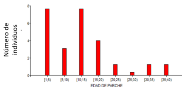
Fig. 2. distribución de P. nigra según la edad del parche ripario.
