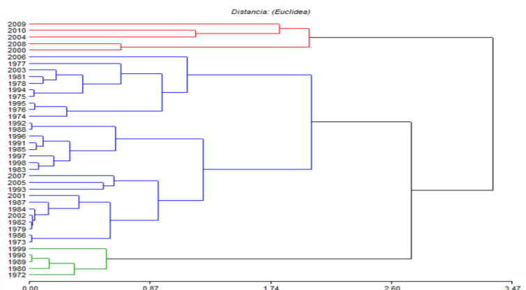
Fig. 4. Relación pulsos del río Limay/Tasa de crecimiento anual de la población de álamos
